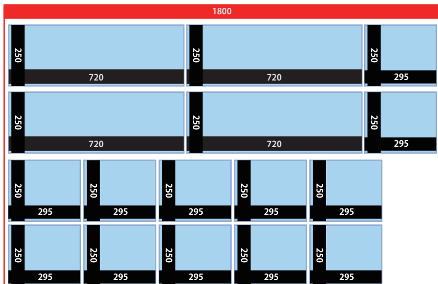
木取り図 (単位 :mm)
