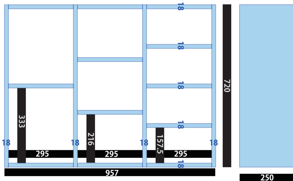
木取り図 (単位 :mm)
